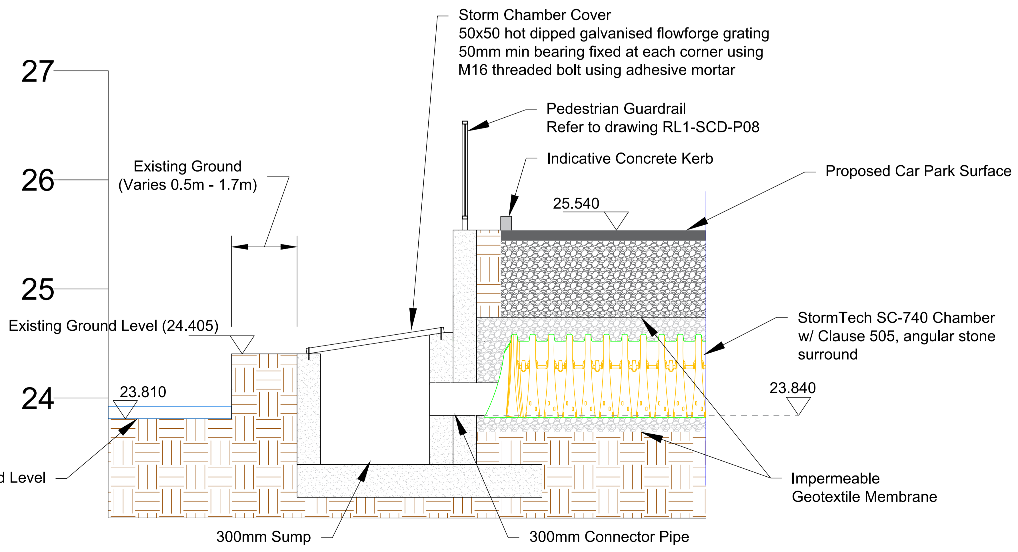
Section A-A
